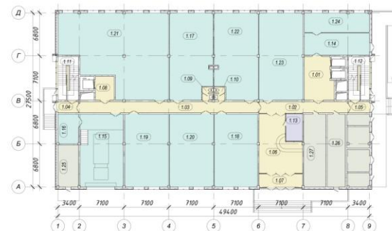
План 1 этажа
